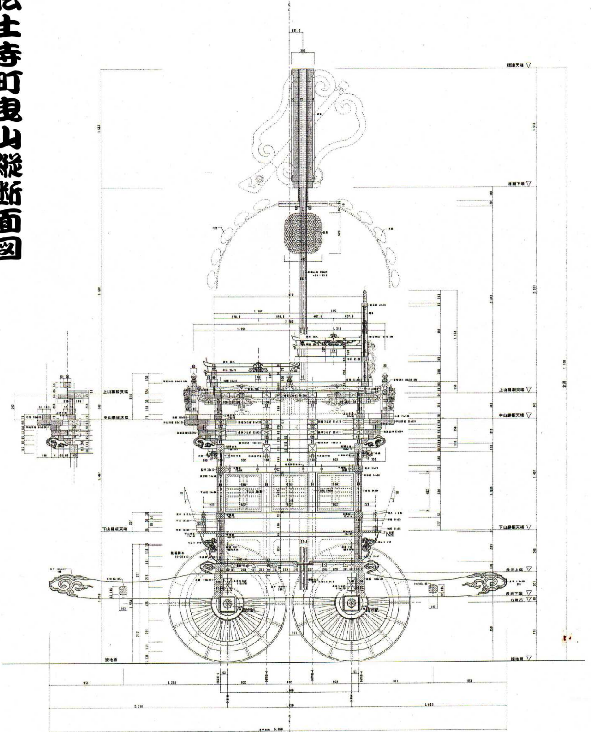
縦断面図
